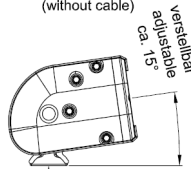
Ansicht von der Seite: (ohne Anschlussleitung) side view (without cable)
