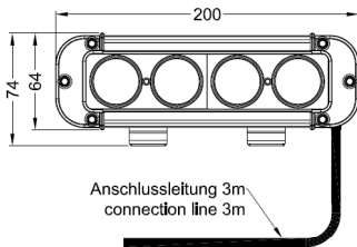
ILED6.40 Ansicht von vorne: front view
