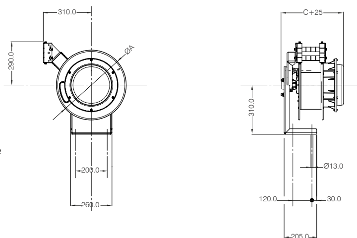
1703 - Upevňovacie zariadenie
